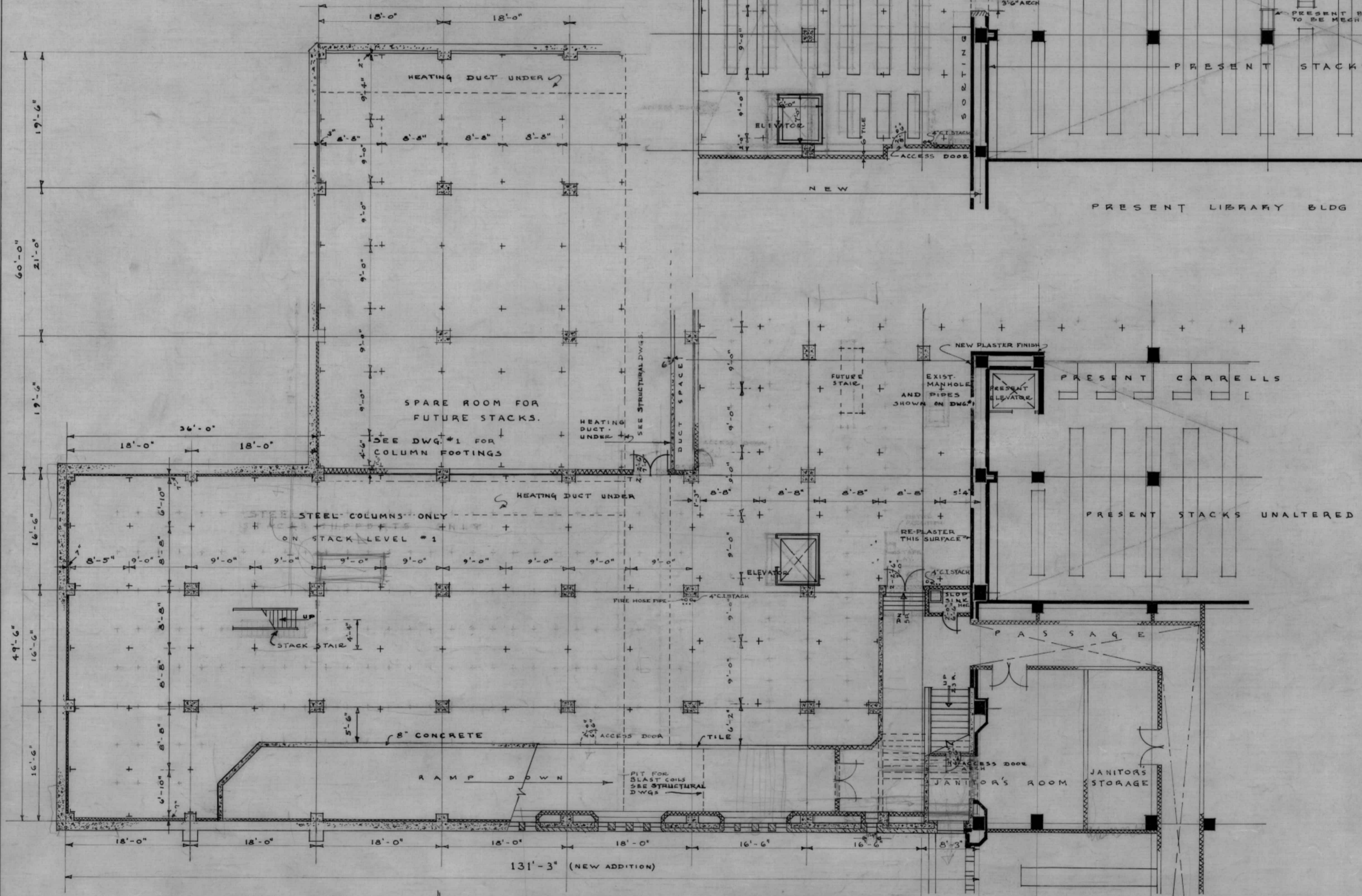
STACK LEVEL #1 SCALE: 1/8" = 1'-0"
